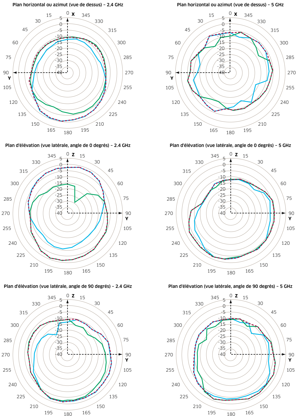
Figure 2. Tracés de modèles d'antenne OmniAccess AP1201
